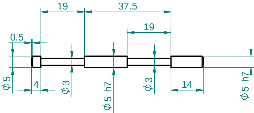
Valvula Vastago (2u) (AISI 316)
