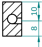
SECTION AG-AG
