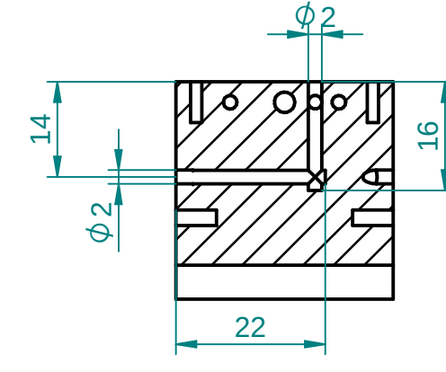
SECTION V-V
