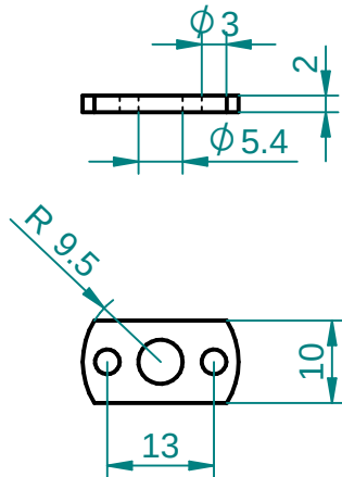
Valvula Agua Tapa Vastago
