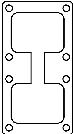
Valvula Caja Junta (0.5mm)(2u)
