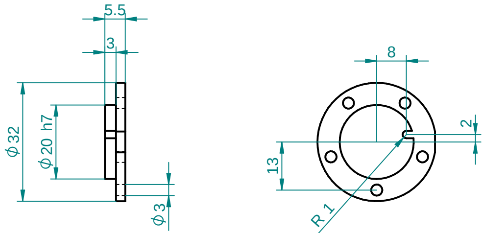
Cilindro Vapor Grueso Tapa Derecha
