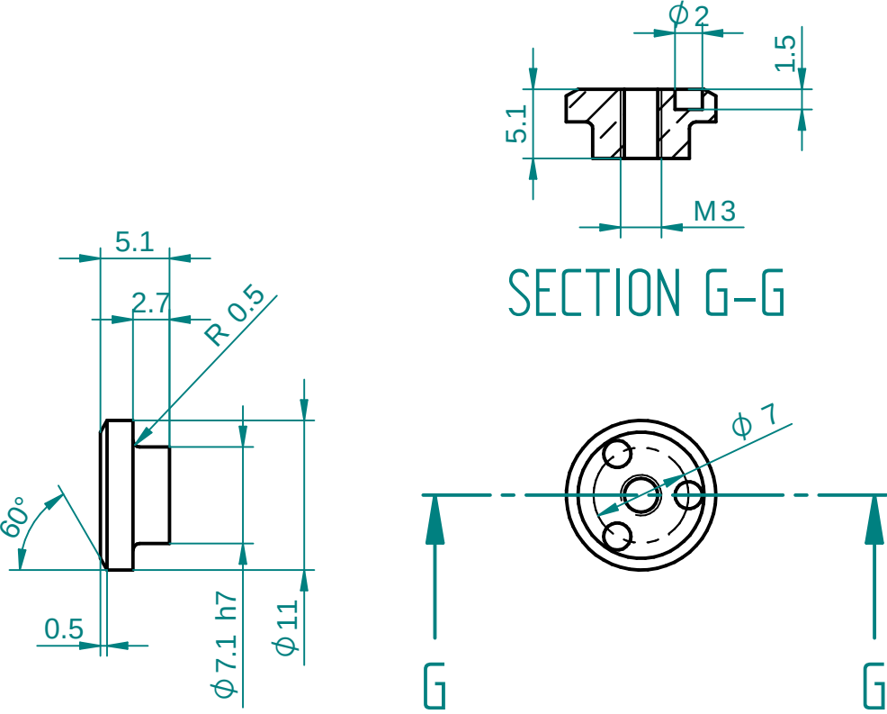
Piston Agua Parte 2 (2u)
