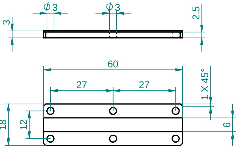
Valvula Agua Tapa Superior
