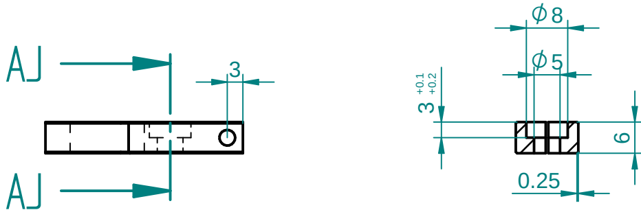
SECTION AJ-AJ
