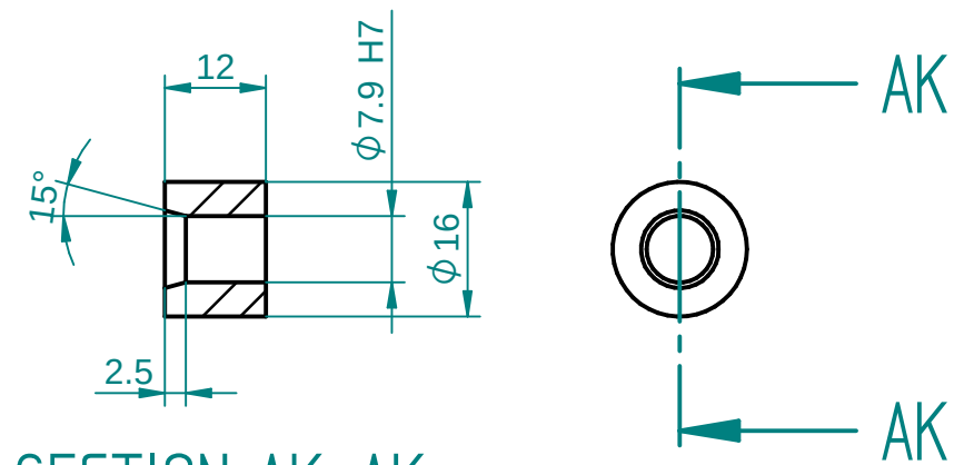
SECTION AK-AK
