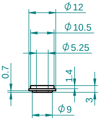
Valvula Agua Asentamiento Bola (8u)
